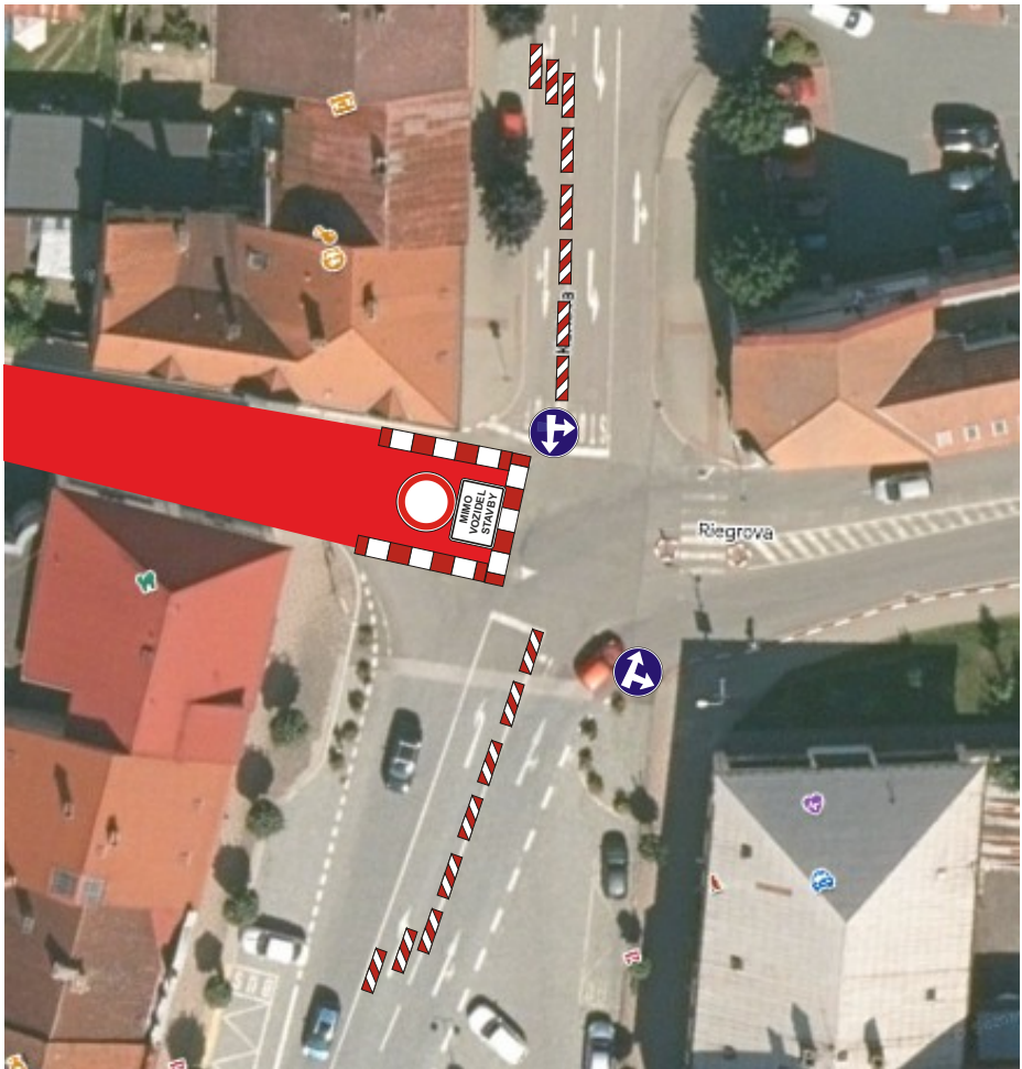
Detail křižovatky II/501 ul. Riegrova a ul. Čsl. armády
